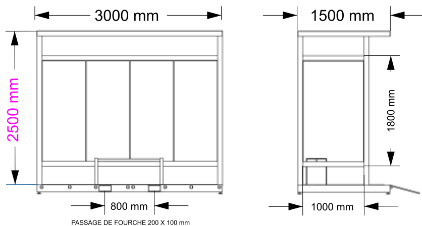
Réf 25°/ABB1-(+ref cloison voir p.2) (version 3x1.5m)
